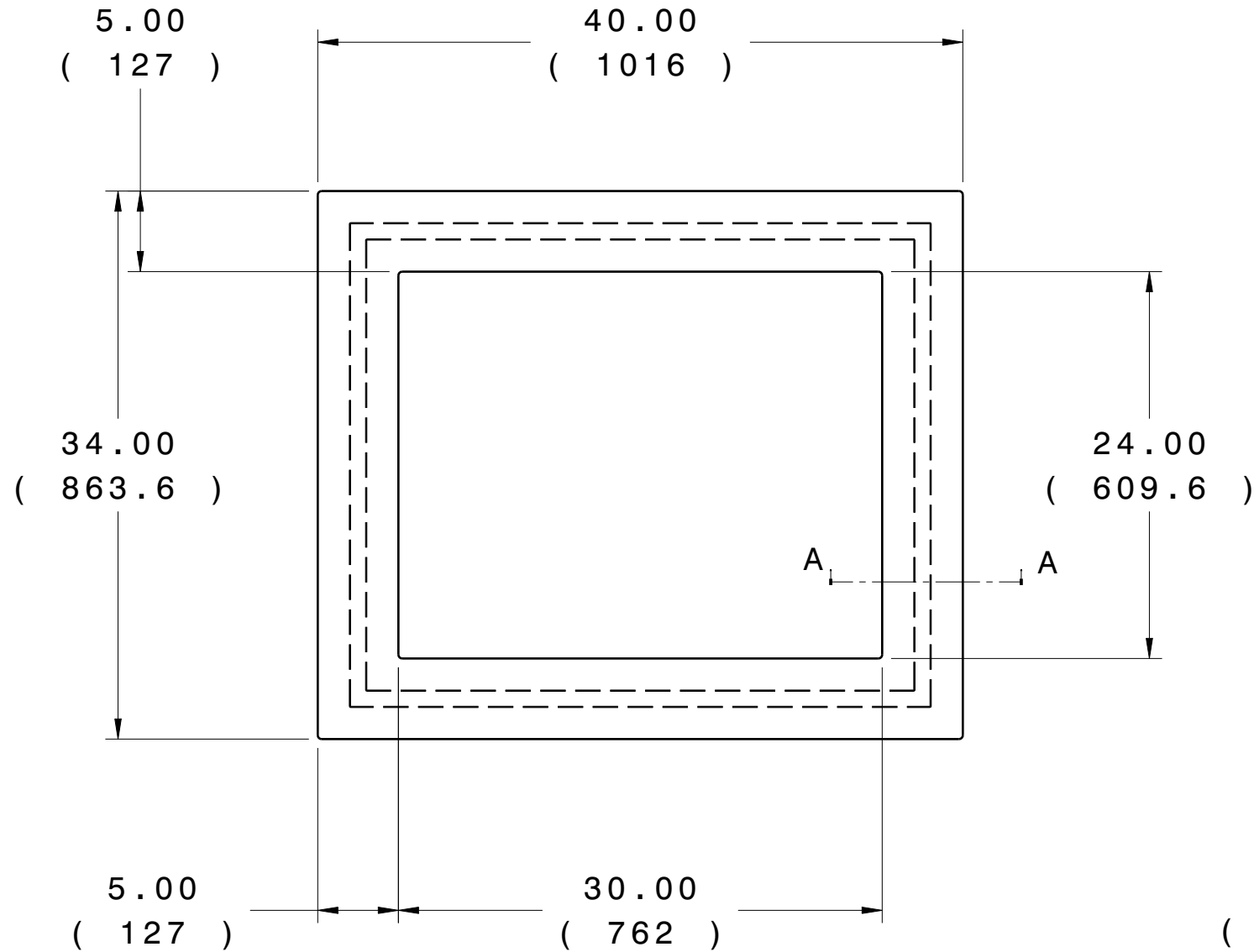
Front view Scale: 1:10
